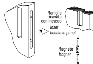
Anta predisposta per magnete e maniglia ricavata con incasso Pre-mortised door (hole) for magnet and inset handle in panel
