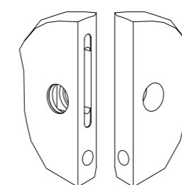
Křídlo připravené s otvorem pro sadu Chiudiscrigno se zámkem nebo s evropskou cylindrickou vložkou
