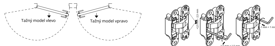
Skryté panty nastavitelné na 3 osách
