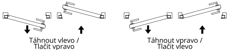
Battente50 komplet pro omítku 105 a více / sádrokarton 100 mm – Táhnout vlevo – Táhnout vpravo – Tlačit vpravo – Tlačit vlevo
