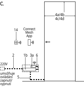
C. Ovládání: zapínání a vypínání pomocí nástěnného tlačítka nebo speciální aplikace.
