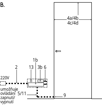
B. Provoz: zapnutí a vypnutí se zavřením/otevřením křídla.
