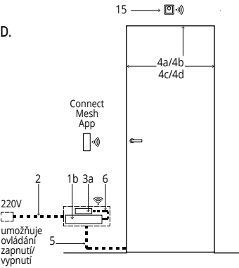
D. Provoz: časované zapnutí (30") prostřednictvím pohybového snímače nebo speciální aplikace.
