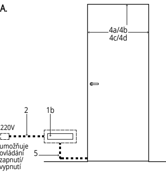
A. Provoz: zapínání a vypínání prostřednictvím zařízení (není součástí dodávky) na hlavní napájení.
