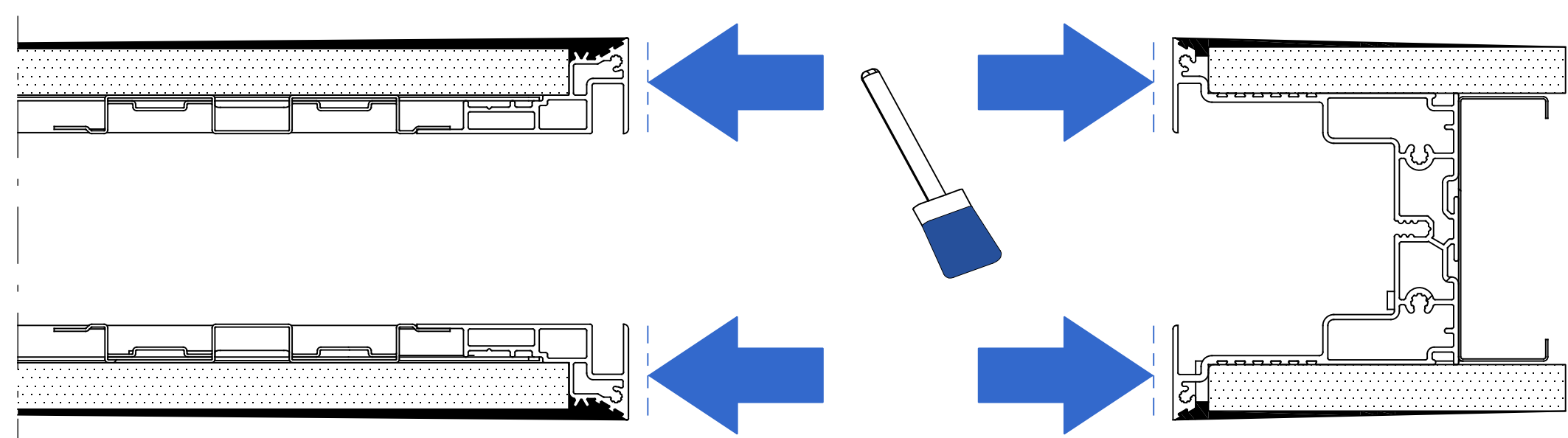
ANTA SINGOLA - PORTE SIMPLE - UNA HOJA EINFLÜGELITE TÜREN - SINGLE DOOR
